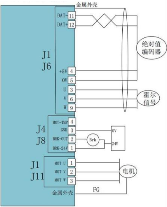
DE2系列驱动器
