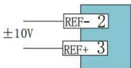
图3.2.2 外部电源模拟量输入接线
